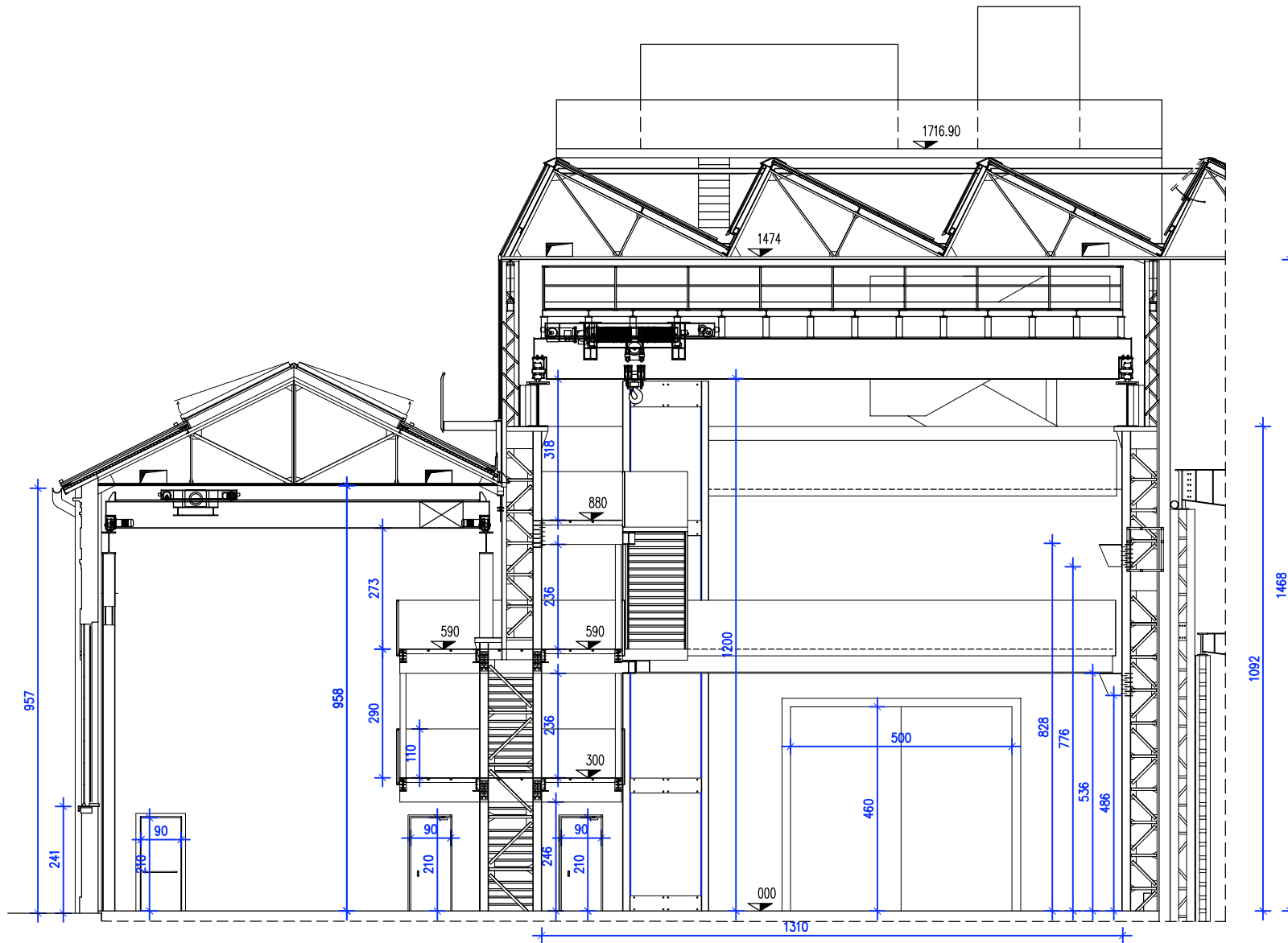
SEZIONE TRASVERSALE A-A
